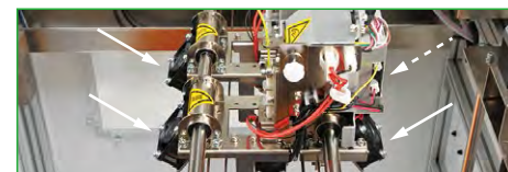
ヘッド前後に2個ずつ搭載された冷却ファン(白矢印)
